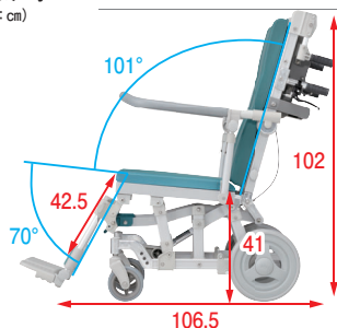
背上げ時 (単位: cm)
