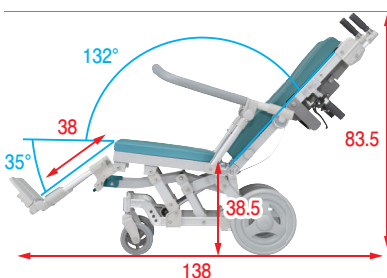
リクライニング時(連動) (単位: cm)
