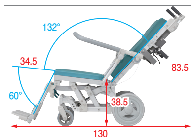
リクライニング時(連動解除) (単位: cm)
