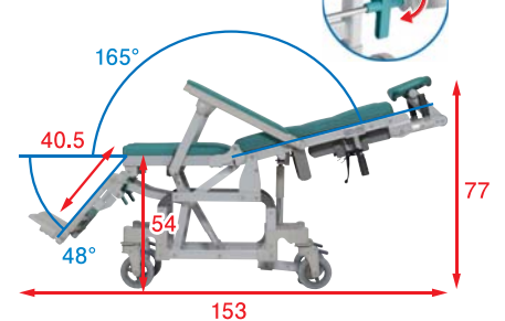
リクライニング時(連動解除)
