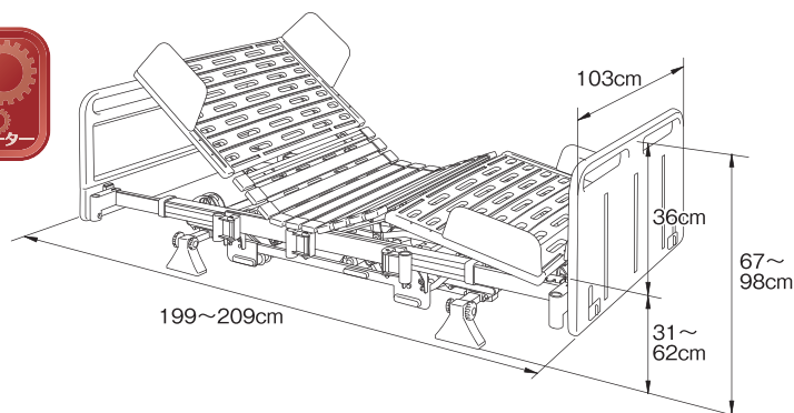
規格図
